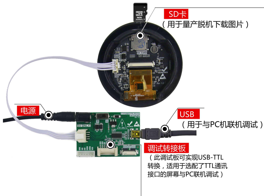
图 1-3 TTL 调试工具图
